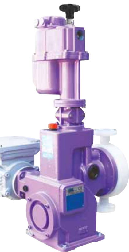
Bomba XL de simple membrana hidráulica con cabezal en PVDF. Regulación automática del caudal mediante servomotor eléctrico , diseñado por OBL, y con protección IP66. Incluye resistencia anticóndensación que le permite trabajar en ambientes difíciles como salino y/o áreas desérticas con altas variaciones de humedad y temperatura.
